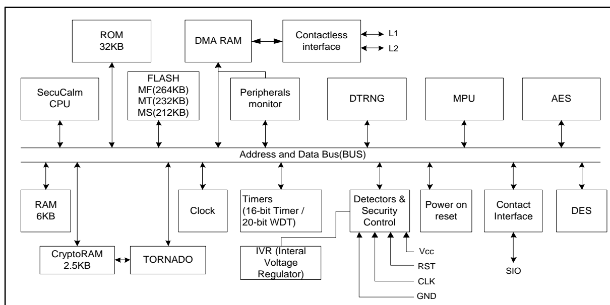
Figure 1 S3FT9ME/S3FT9MT/S3FT9MS Block Diagram
