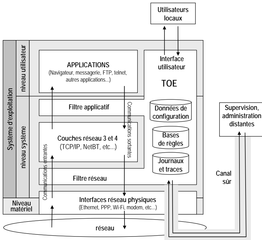
Figure 3 : schéma d'architecture de la TOE
