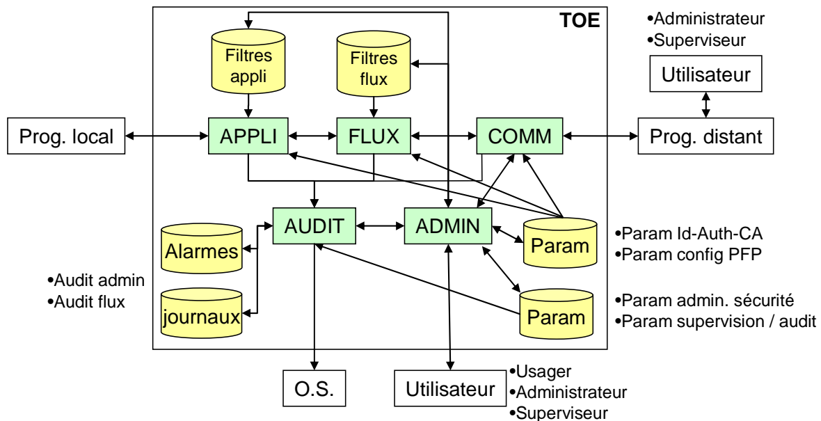
Figure 2 : modélisation de la TOE et de son environnement
