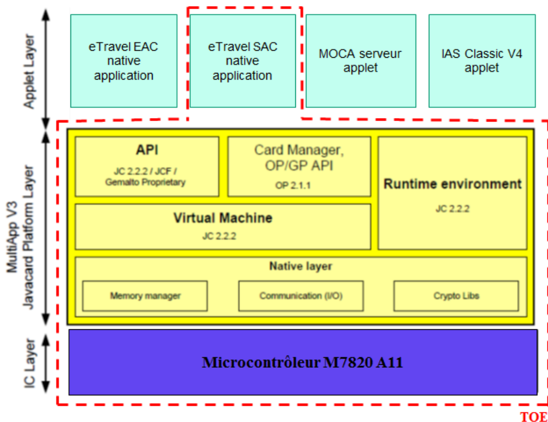
Figure 1 - Architecture et périmètre de la TOE
