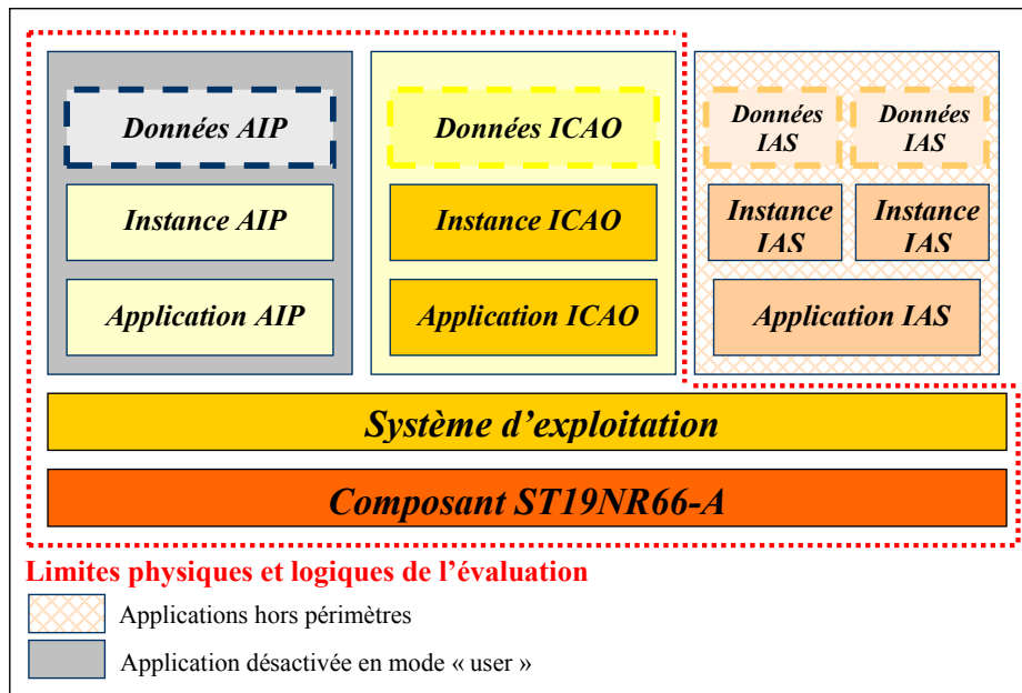
Figure 1 – Architecture du produit
